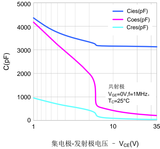
图7. 电容特性
