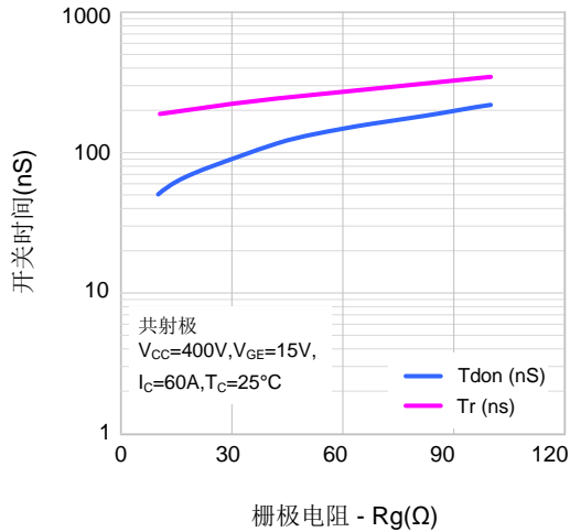
图9. 开启特性 vs. 栅极电阻
