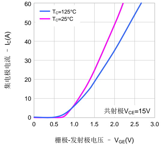
图2. 传输特性
