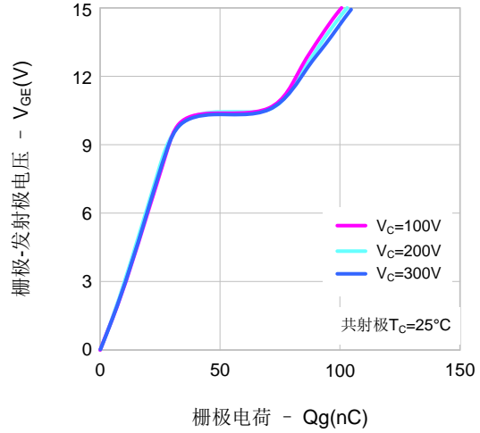
图8. 栅极电荷
