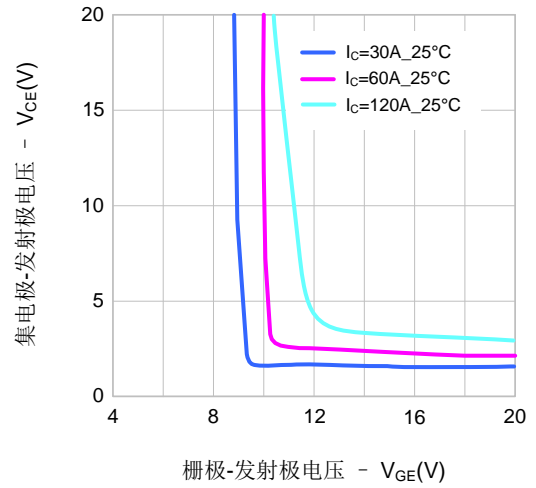
图4. 饱和电压 vs. 栅极-发射极电压
